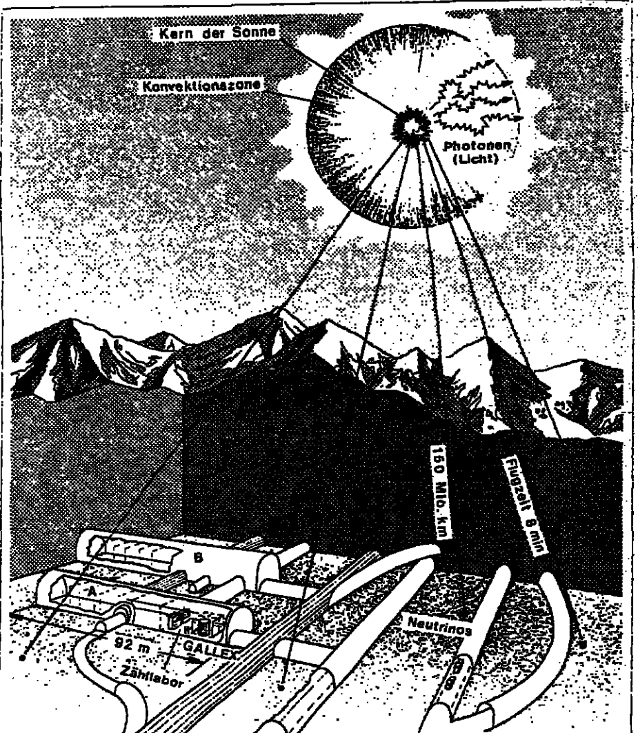
Schematische Zeichnung des europäischen Untergrundlabors unter dem Gran Sasso-Bergmassiv: In einem Teil der bereits vollständig ausgeschachteten Halle A wollen Wissenschaftler mit einem aus 30 Tonnen Gallium-Chlorid bestehenden Detektor von der Sonne kommende Neutrinos messen. Grafik: MPG/SCHÄFER
